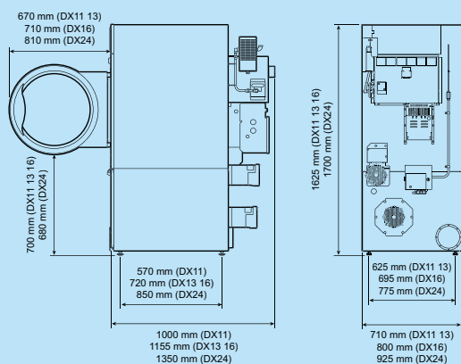
Seitenansicht DX 11 13 16 24
